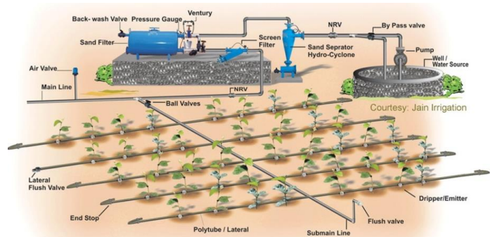
Das Tropfenbewässerungssystem
